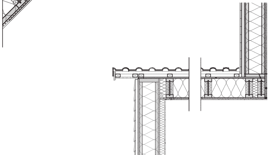
Ortgang und Gaubenanschluss
